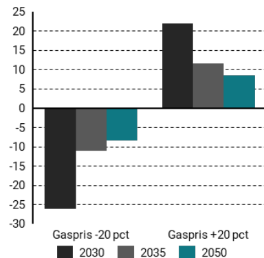
Figur 18.3 Gasprisfølsomhed på elpriser i forhold til grundforløbet (DKK/MWh)
