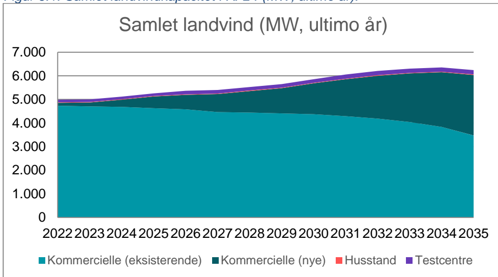
Figur 6.1: Samlet landvindkapacitet i KF24 (MW, ultimo år).
