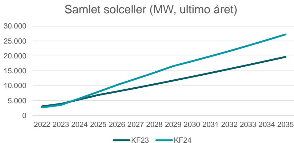
Figur 7.3: Samlet solcellekapacitet i KF23 og KF24 (MW)
