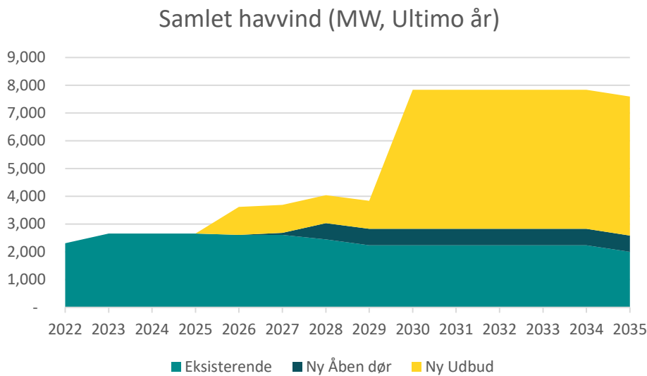
Figur 5.1: Samlet kapacitet for havvind i KF24 (MW).
