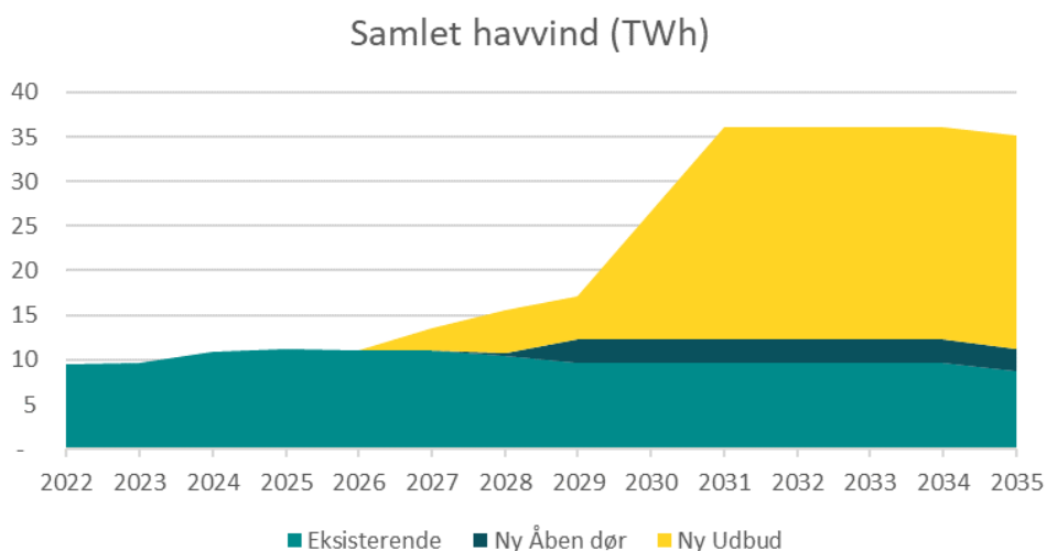
Figur 5.2: Samlet produktion for havvind i KF24 (TWh).
