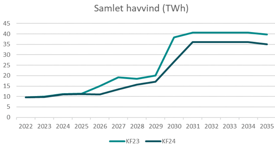
Figur 5.4: Samlet produktion fra havvind i KF23 og KF24 (TWh).
