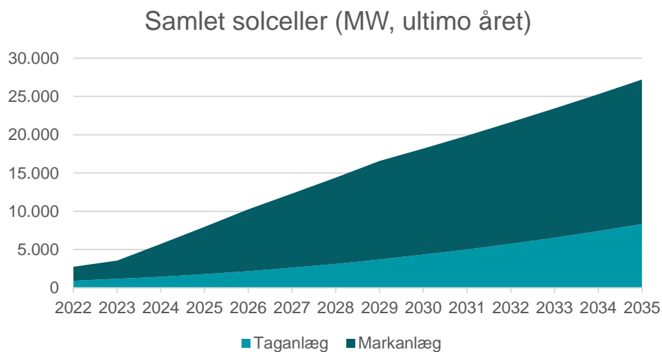
Figur 7.1: Samlet solcellekapacitet i KF24 (MW, ultimo året)
