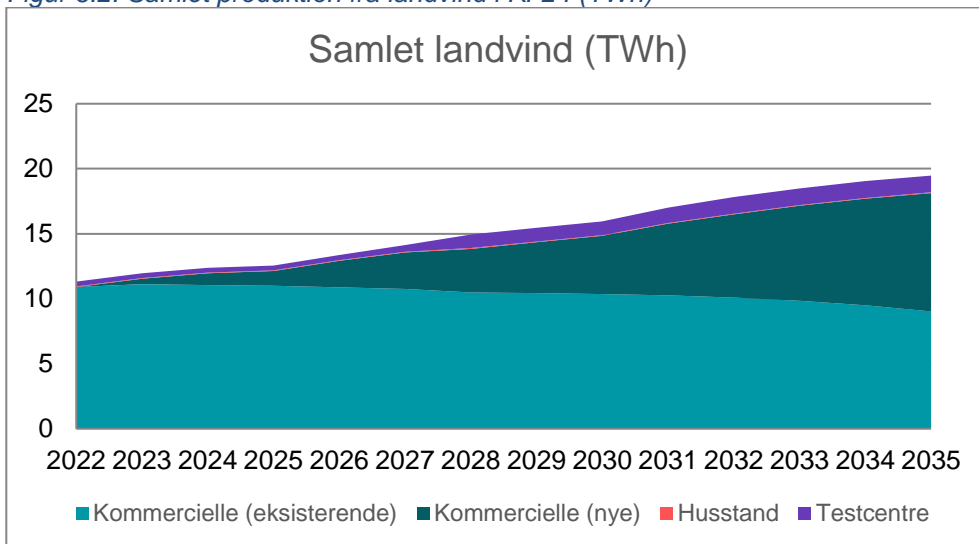
Figur 6.2: Samlet produktion fra landvind i KF24 (TWh)
