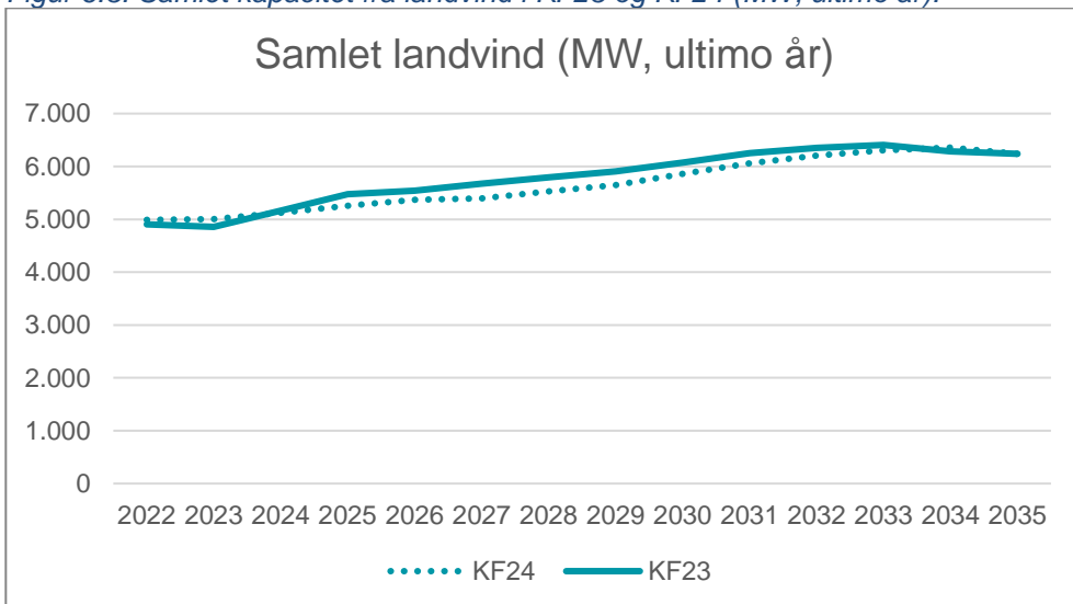
Figur 6.3: Samlet kapacitet fra landvind i KF23 og KF24 (MW, ultimo år).
